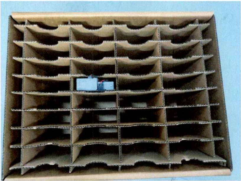
图二，将 9 个长刀卡和 5 个短刀卡如图所示进行组装，一箱一层，一层 32PCS。注意将 PA03865 的线材放入格子内
